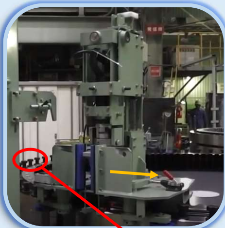
①ボルト位置へ移動
