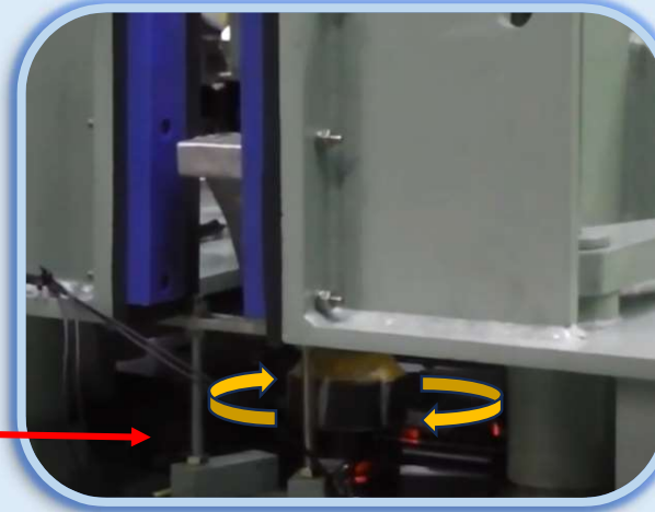
③設定トルクで締付後、次のボルトへ移動
